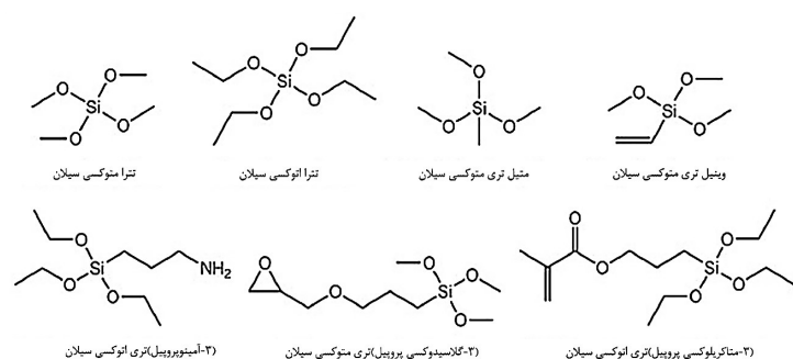
شکل ۳. ساختار مولکولی تعدادی از آلیکوسی سیلان های پر کاربرد مانند تترااتوکسی سیلان، تترااتوکسی سیلان، متیل تری متوکسی سیلان و... (Kudryavtsev & Figovsky, 2015)
