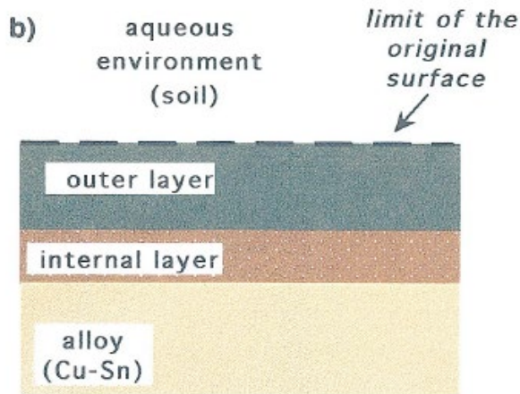
شکل ۱. طرح شماتیک لایه‌ها در پاتین نوع (۱) (Robbiola & et al, 1998) Figure 1. Schematic diagram of the layers in type (1) patina (Robbiola & et al, 1998)
