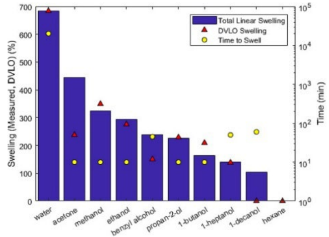
شکل ۸. نمودار میزان تورم اتفاق افتاده در ذرات رس موجود داخل آجر در مقابل حامل های مختلف (Erdogan et al., 2023).
