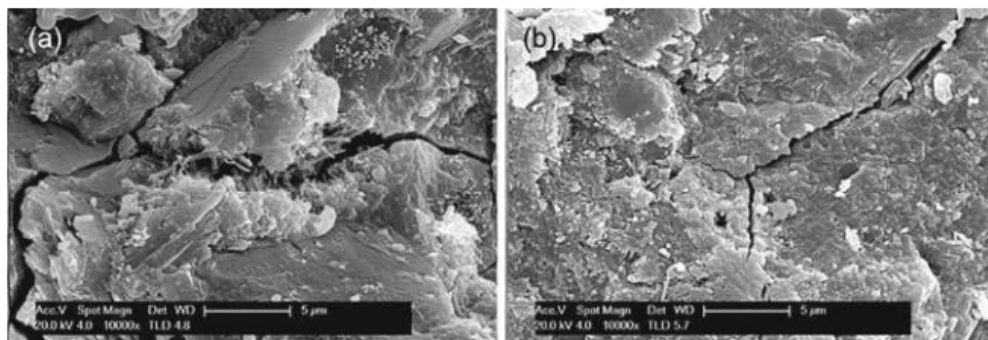
شکل ۶ تصاویر SEM از نمونه تحت درمان سمت چپ: اعمال در مرحله ابتدایی و سمت راست: درمان با اکسید گرافن پس از ۲۸ روز از گیرش (Faria et al., 2017)
