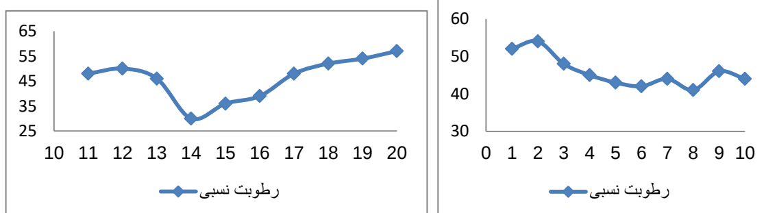
شکل ۳۲: نمودار رطوبت نسبی در محیط سالن نمایش موزه (تاریخ ۱۰ تا ۲۰ آذر) (منبع: نگارنده)
