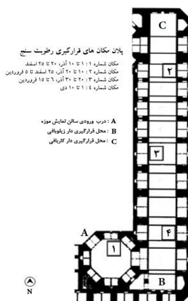
شکل ۳۱: پلان نقاط سنجش رطوبت نسبی و درجه حرارت در سالن نمایش موزه (منبع: نگارنده)
