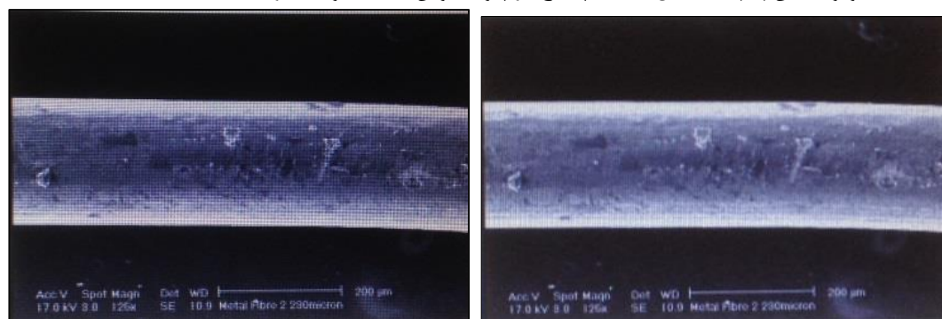
شکل ۴- عکس میکروسکوپی-الف) لیف فلزی نقره ب) لیف فلزی نقره باروکش طلا SEM
