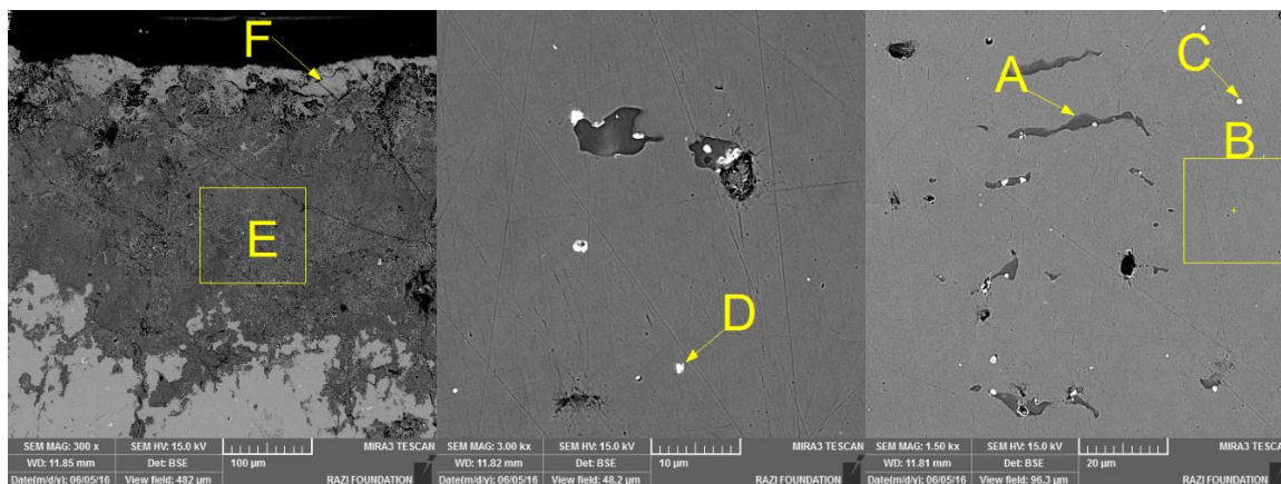
شکل ۱. سمت راست: نقاط A، ناحیه B و نقطه C در آزمون SEM-EDS؛ نقطه D: نمونه از جداره ظرف است؛ سمت چپ: ناحیه E و نقطه F، نمونه از جداره ظرف است (منبع: نگارنده)
