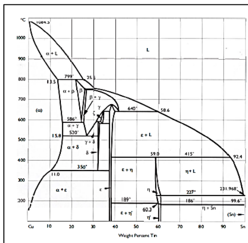
شکل ۱۴. نمودار فازی مس - قلع (Scott, 1991, p. 122)
