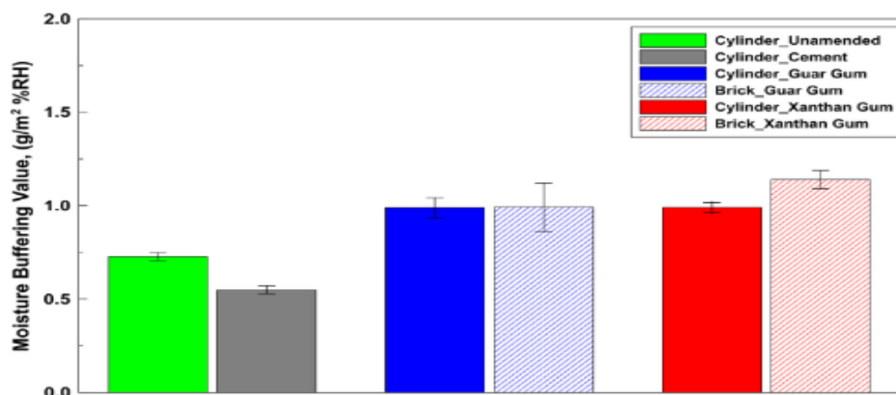
شکل ۳. مقادیر جذب رطوبت برای تمام نمونه‌ها (Muguda-Viswanath, 2019)
