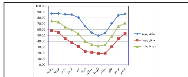
شکل ۹. نمودار میانگین حداکثر، حداقل و متوسط رطوبت نسبی ماهانه دوره آماری (۱۹۹۰-۲۰۲۳) برحسب درصد.
