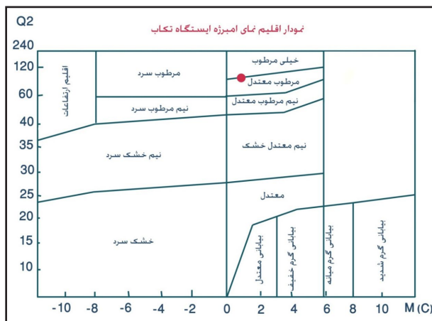
شکل ۱۱. نمودار اقلیم نمای آمبرژه ایستگاه تکاب (قدری، ۶۲: ۱۳۸۸) Fig 11. The ambrothermic climate diagram of the Takab meteorological station (Ghadri, 2009: 62)
